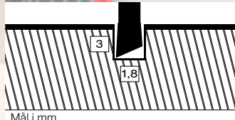
Forridser-snittet
